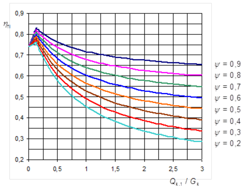
Kuva 1. Pienennystekijän, \eta_{fi} , vaihtelu määrävän muuttuvan kuorman ja pysyvän kuorman ominaisarvojen kuormasuhteen Q_{k,1} / G_k funktiona standardia SFS-EN 1990 koskevassa ympäristöministeriön asetuksessa esitettyjen kuormien yhdistelysääntöjen mukaan.
