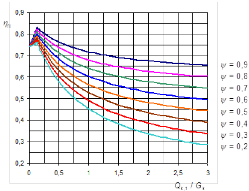
Figur 1. Variation av reduktionsfaktorn \eta_{fi} beroende på lastförhållandet Q_{k,1} / G_k mellan de karakteristiska värdena för den dimensionerande variabla lasten och den permanenta lasten baserat på kombinationsreglerna för laster enligt miljöministeriets förordning gällande standard SFS-EN 1990.
